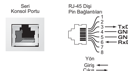
Şekil 5 Seri Port Pin Bağlantıları
