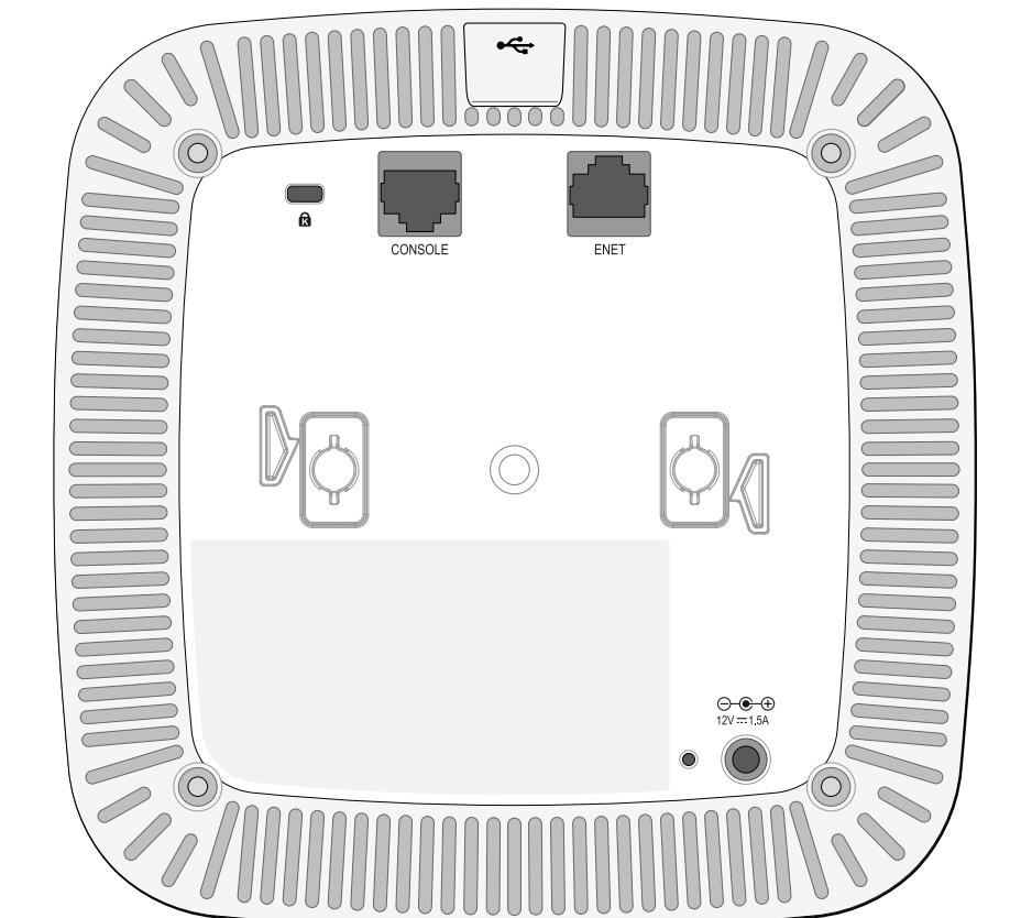
Şekil 4 W-AP210 Serisi Alttan Görünüm
